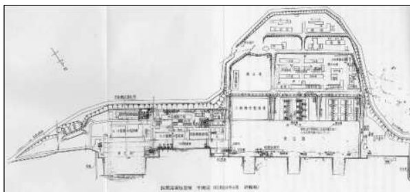
詫間海軍航空隊基地の平面図
