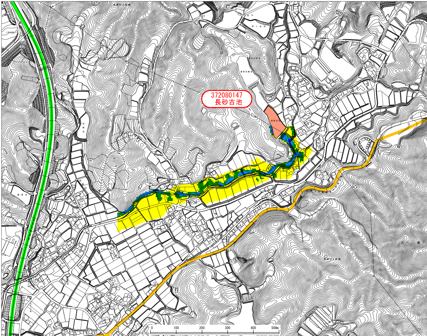
三豊市ため池氾濫解析 浸水想定区域図 (最大浸水深)
