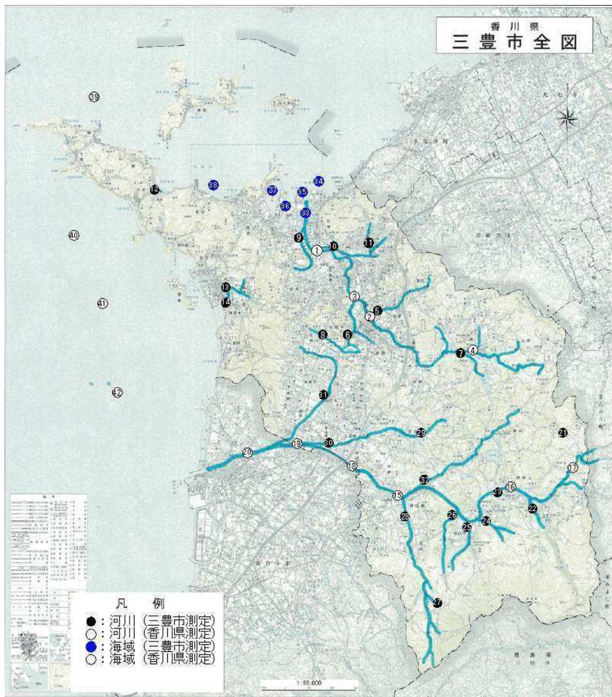
図 3-1-2 三豊市及び周辺海域の公共用水域水質及び底質測定地点
