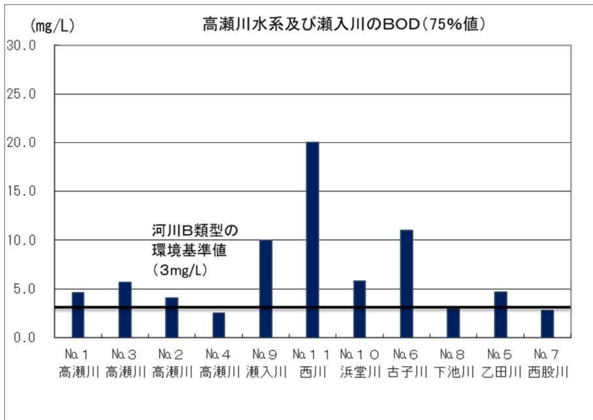
図 3-1-3 高瀬川水系及び瀬入川のBOD
