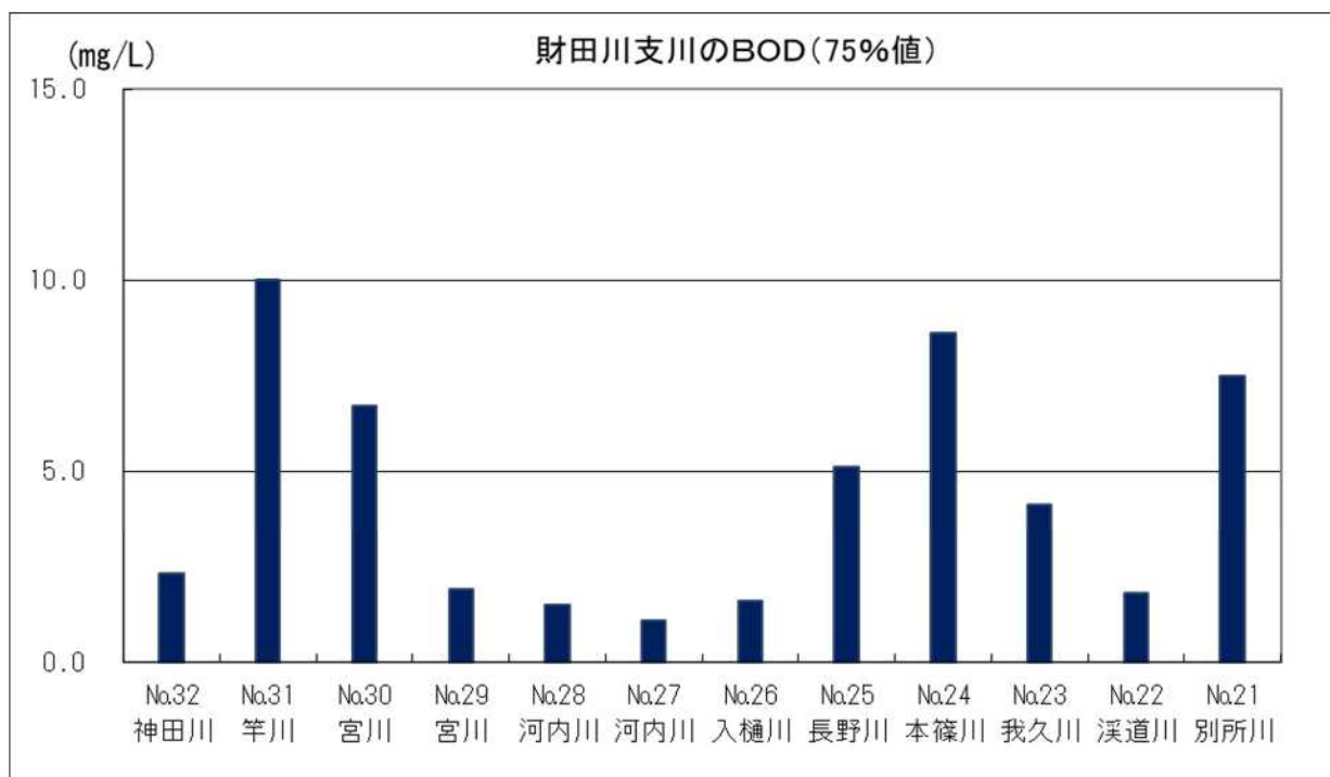
図 3-1-6 財田川支川のBOD
