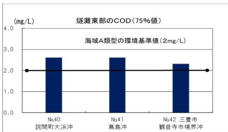
図3-1-8 燧灘東部のCOD
